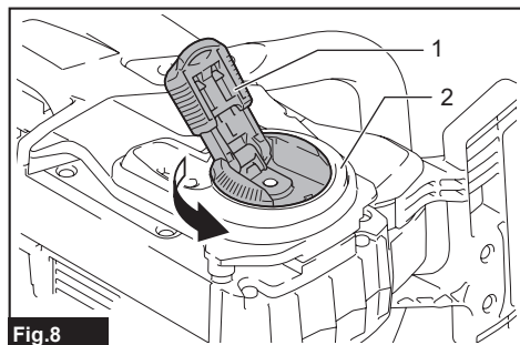
Fig. 8 ► 1. Lever 2. Sprocket cover
